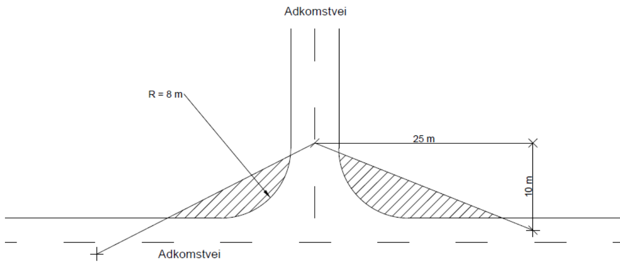
Figur 15 Frisikt Adkomstvei – Adkomstvei med 30km/t
