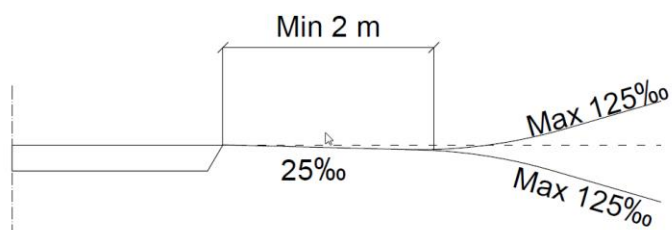
Figur 17 Stigning Avkjørsel – Offentlig vei
