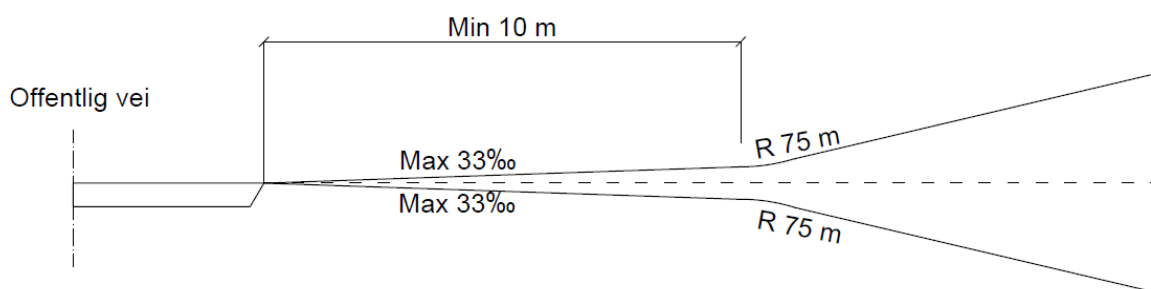
Figur 19 Stigning Adkomst vei II og III
