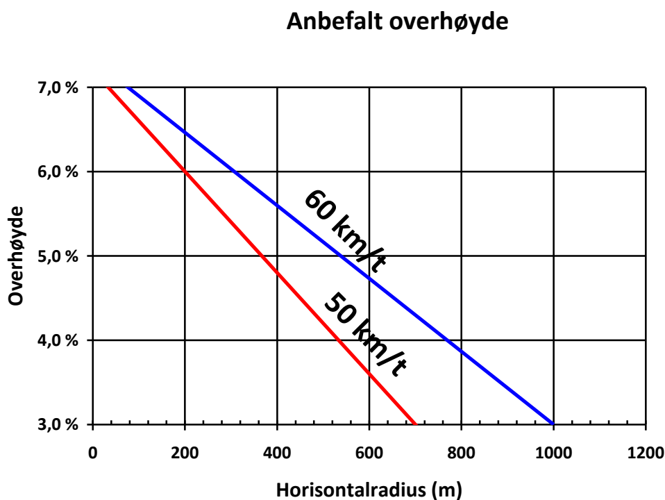
Figur 10 Anbefalt overhøyde
