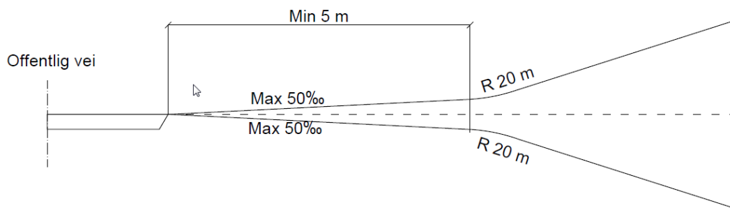
Figur 18 Stigning Adkomstvei - G/S vei
