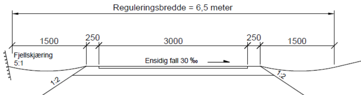
Figur 2 G/S-vei
