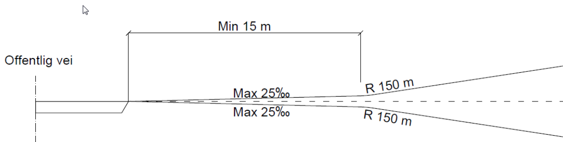
Figur 20 Stigning Samlevei
