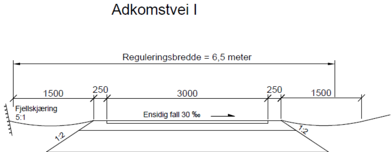
Figur 4 Adkomstvei I
