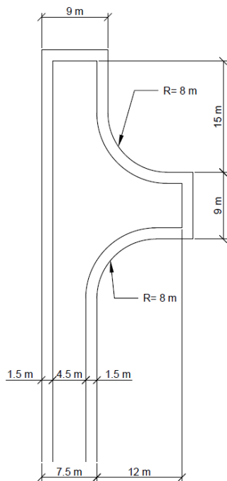
Figur 22 Snuhammer (L)
