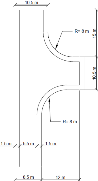
Figur 23 Snuplass (B)
