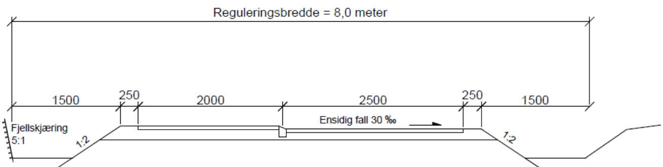
Figur 3 Sykkelvei med fortau
