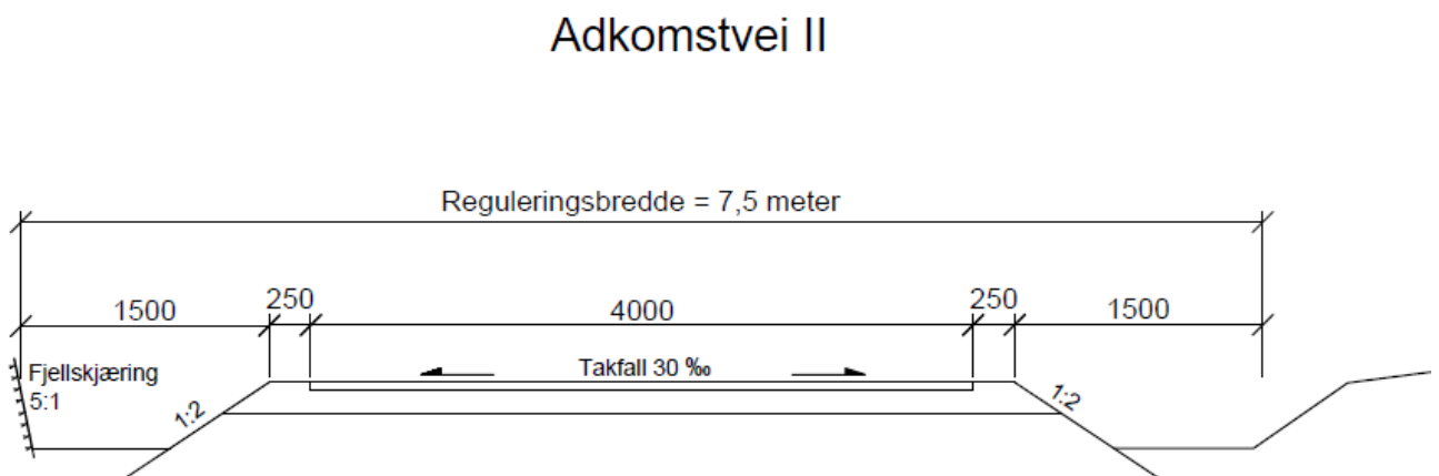
Figur 5 Adkomstvei II
