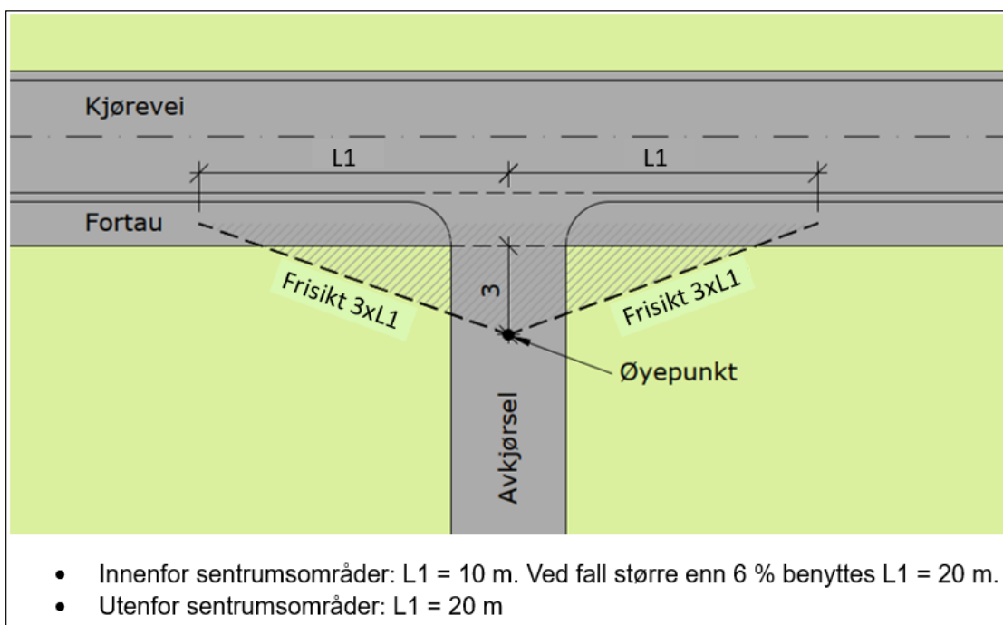
Figur 8: Krav til frisikt der avkjørsel ( \dot{A}DT < 50 ) krysser fortau. Avstand 3 m måles fra asfaltkant på fortau.
