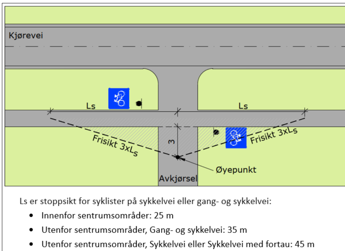
Figur 7: Krav til frisikt der avkjørsel ( \text{ÅDT} < 50 ) krysser sykkelvei eller gang- og sykkelvei. Avstand 3 m måles fra asfaltkant på gang- og sykkelvei.
