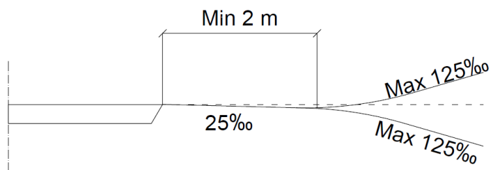
Figur 2 Stigning Avkjørsel - Offentlig vei
